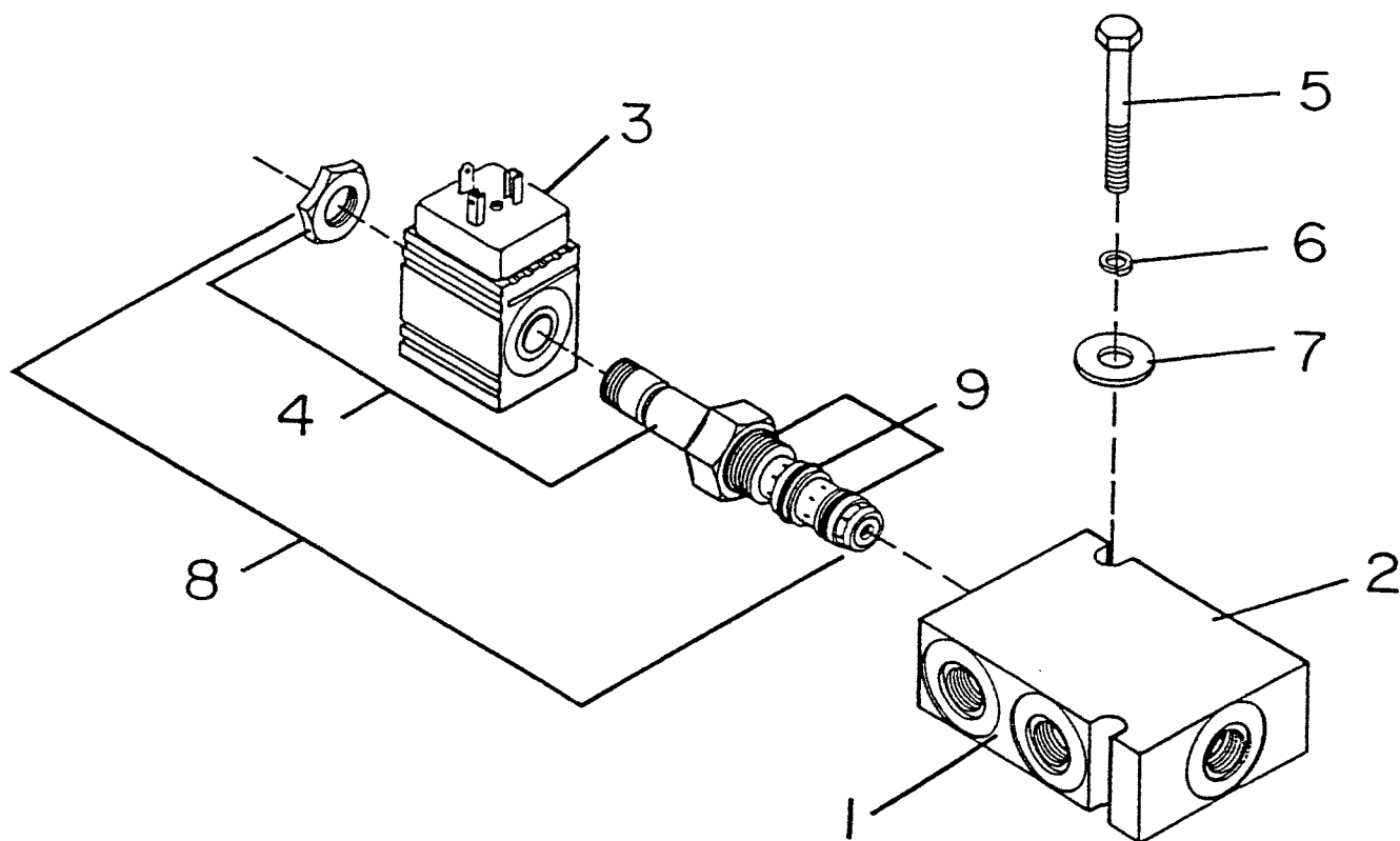
ASSEMBLY ITEMS 2,3,4
